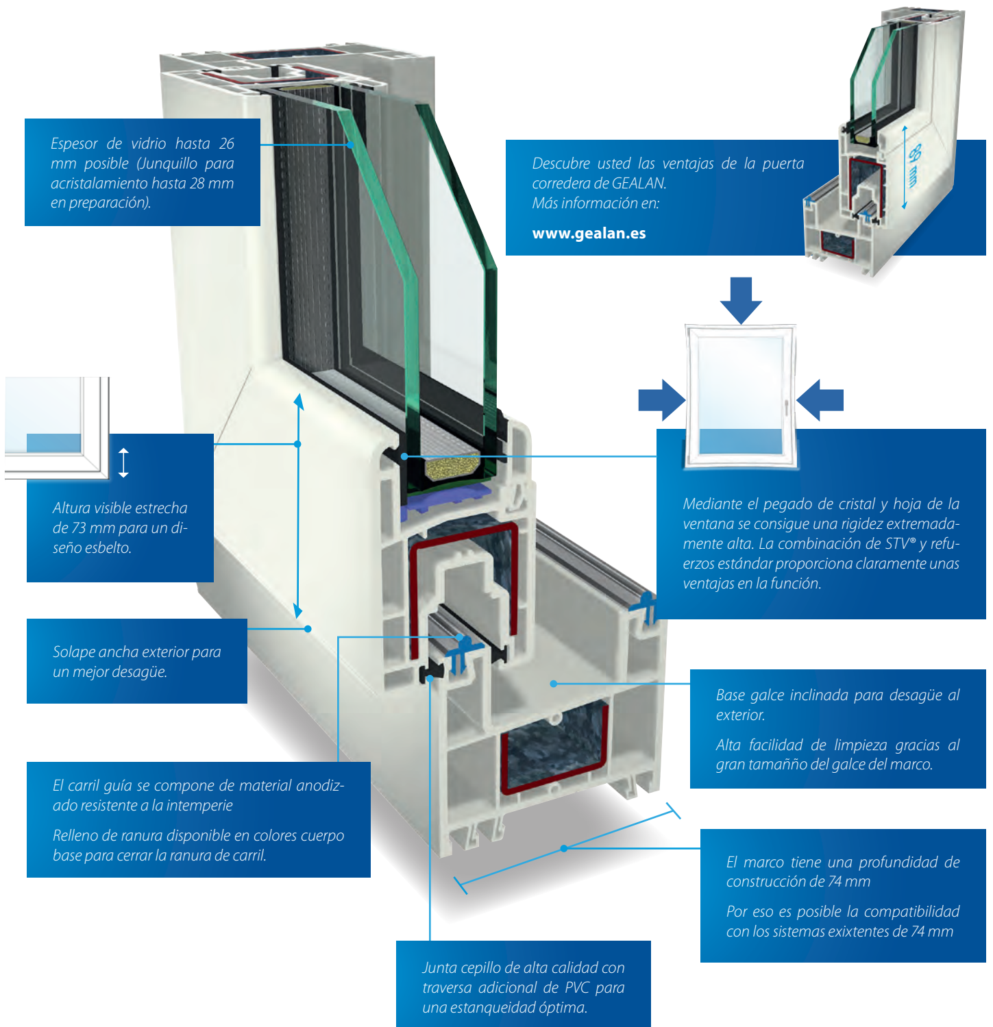
Esquema F
